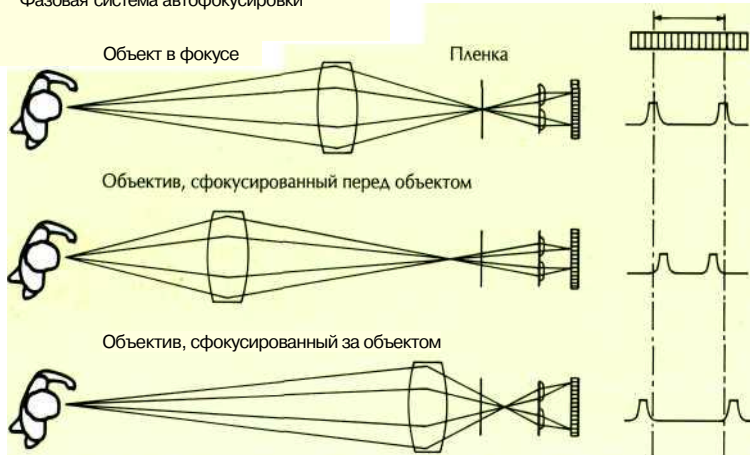
Фазовая система автофокусировки
