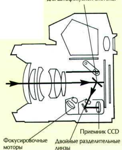
Вспомогательное зеркало для автофокусной системы
